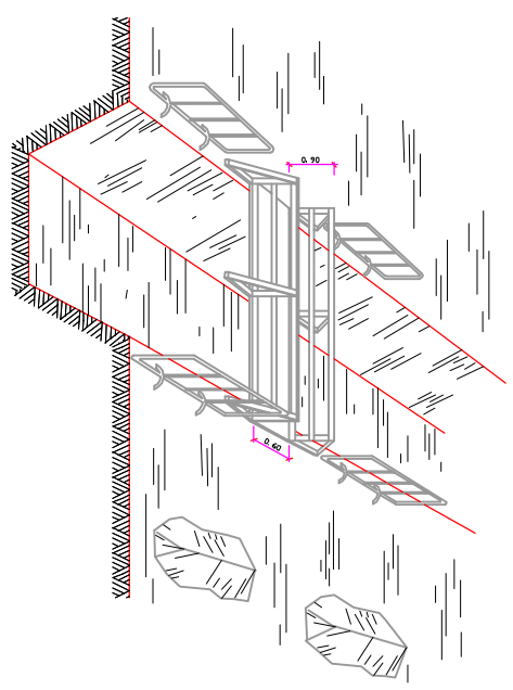
Esquema de protecció de rasos
