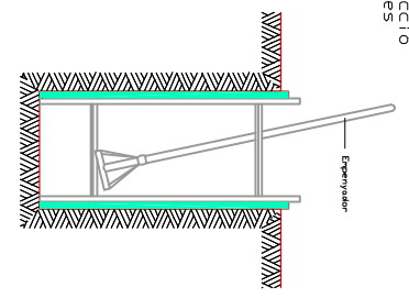
Esquema de protecció de rasos
