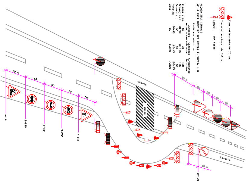
Senyalització en tallis de carrers amb desviament
